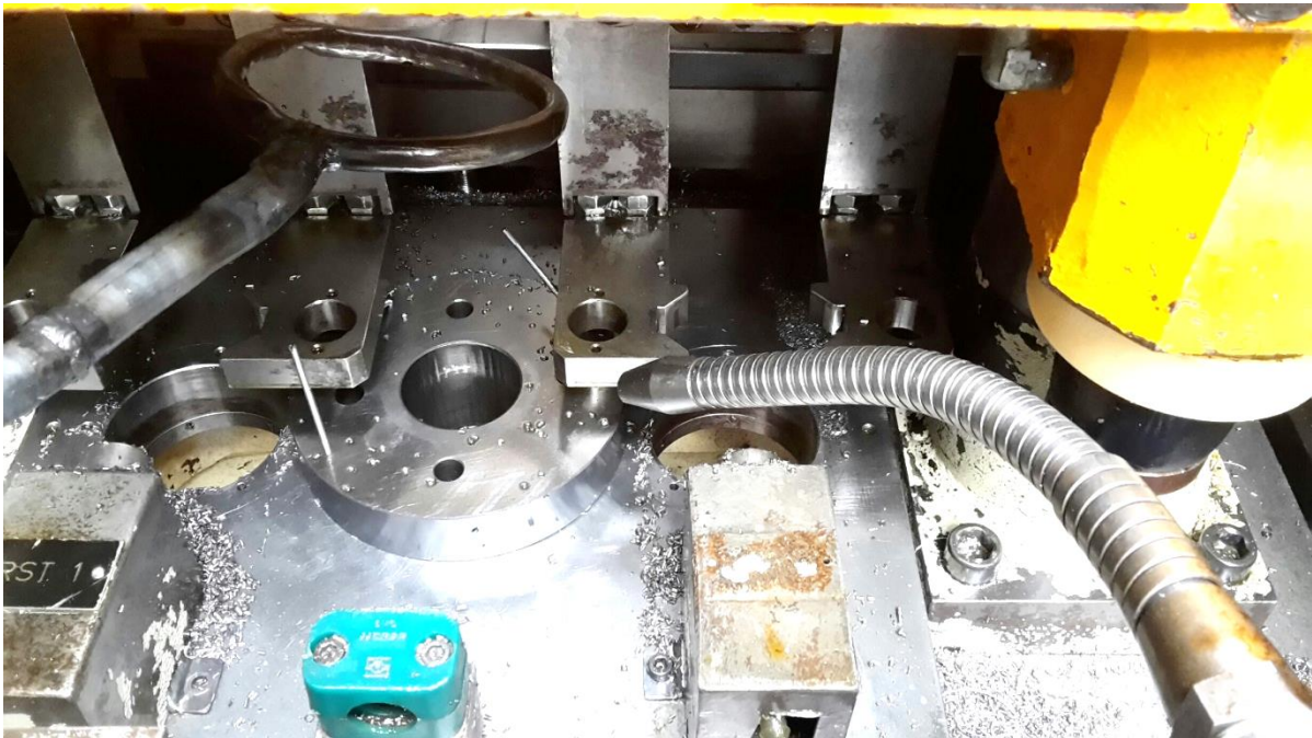
Werkstücktisch mit Werkstückgreifer für 2 Werkstücke Ansicht von der Maschinen Innenseite (vorderseitig)
