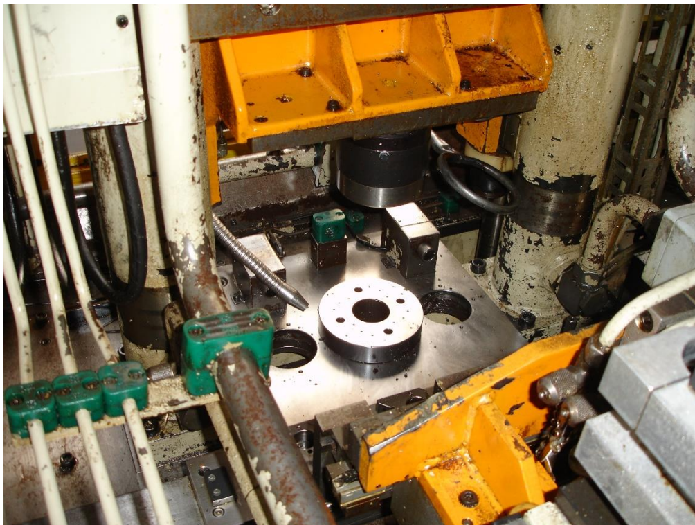
Werkstücktisch für 3 Räumstellen (z.Zt. 2 automatisiert genutzte Räumstellen) Ansicht von der Maschinen- Innenrückseite
