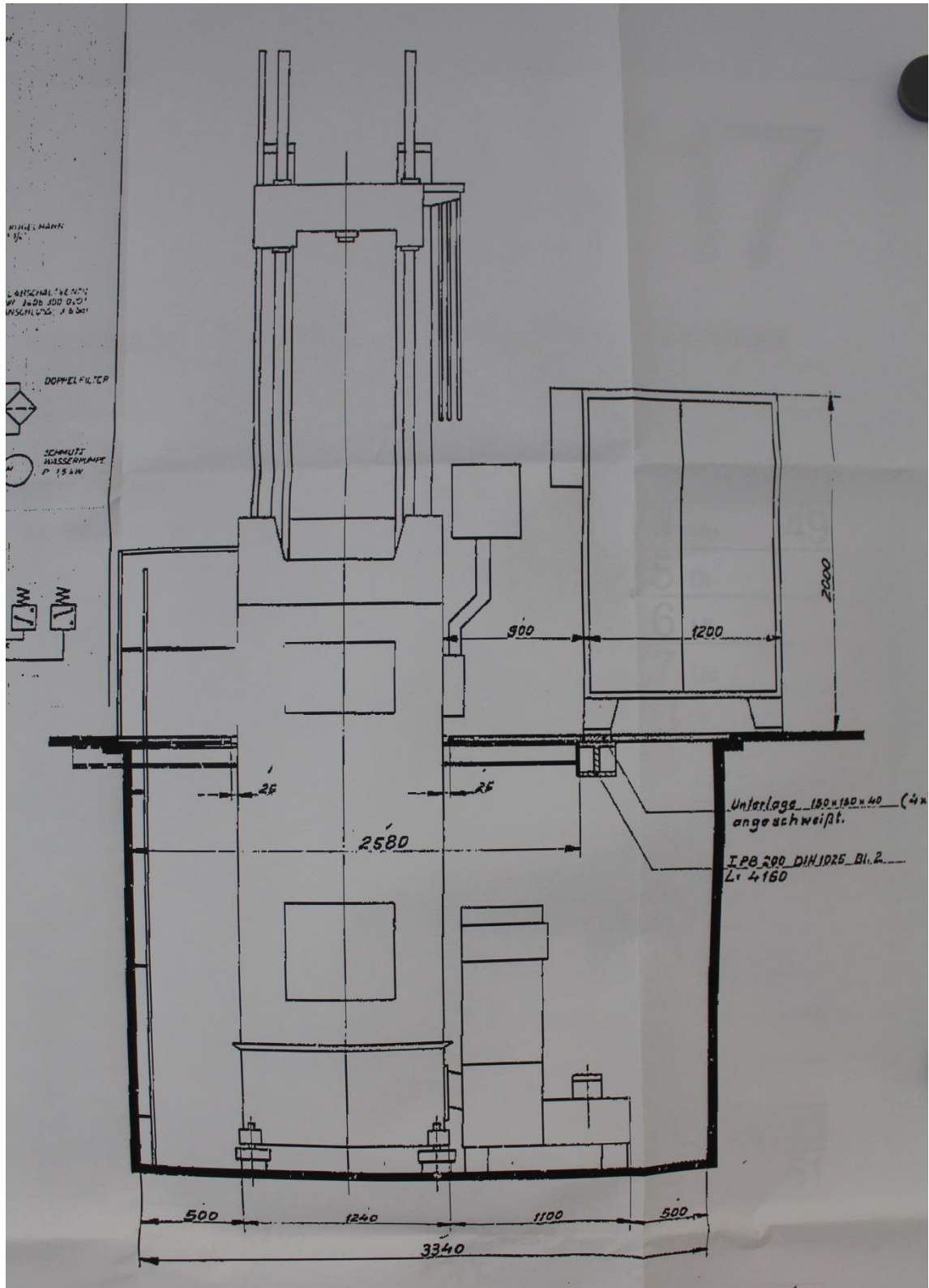
Vorderseitenansicht Maschinenaufstellplan
