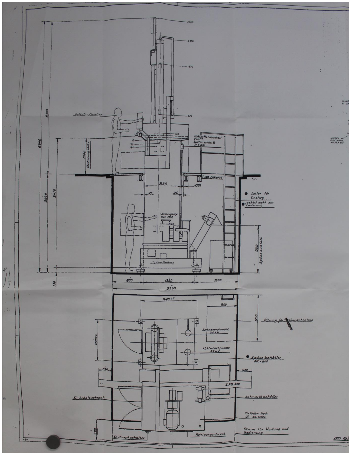
Seitenansicht & Draufsicht Maschinenaufstellplan
