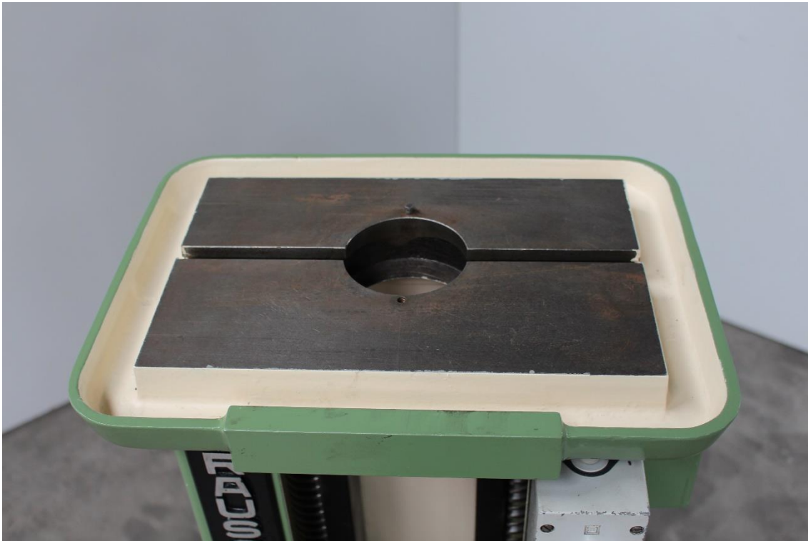
Maschinentisch mit \varnothing 90mm Aufnahme für Räumdorne
