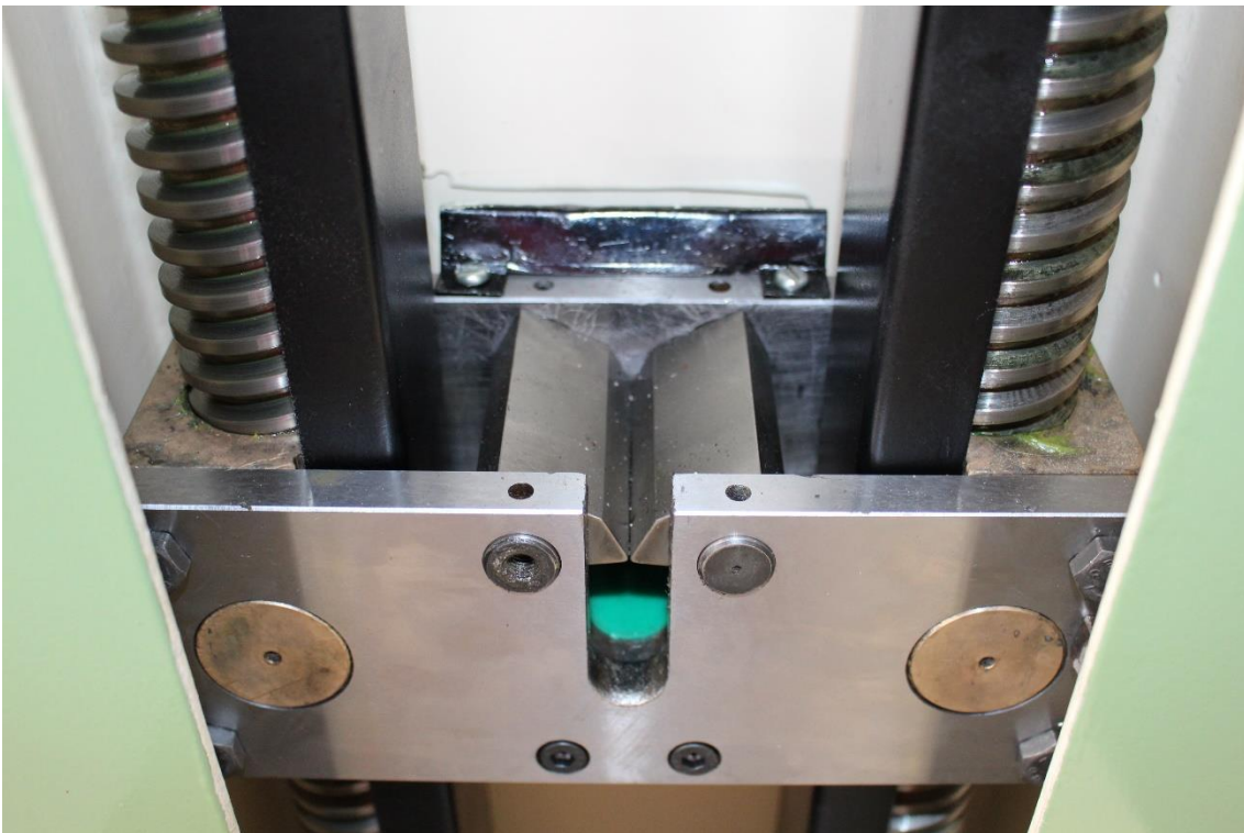
Universal Spannbacken- Ziehkopf für Flachsäfte (überholt und neu justiert)
