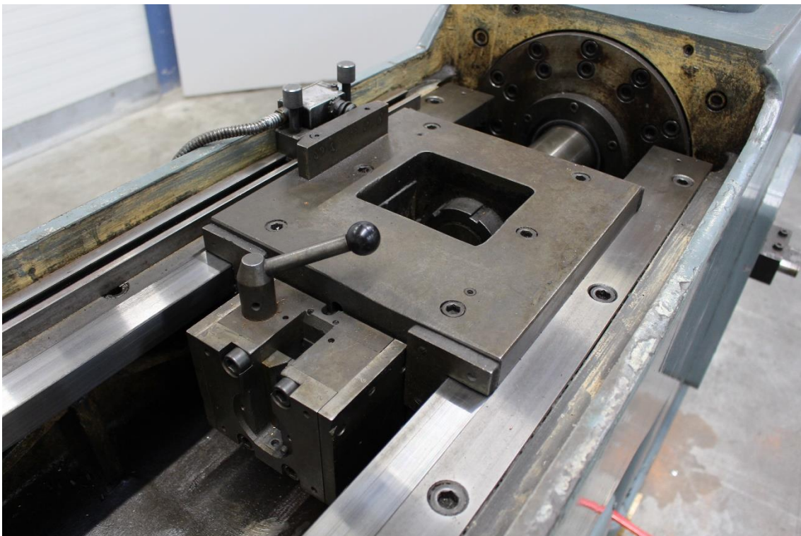
Zugbrücke mit Ziehkopf für Flachsäfte
