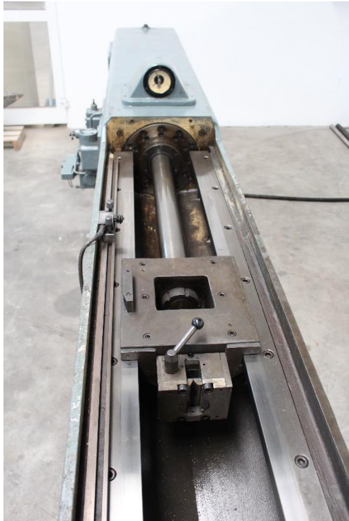
Zugbrücke mit Ziehkopf &amp; Zugkraftanzeige
