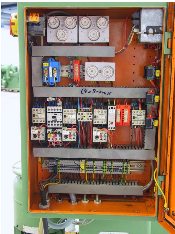
Elektro-Schaltschrank
