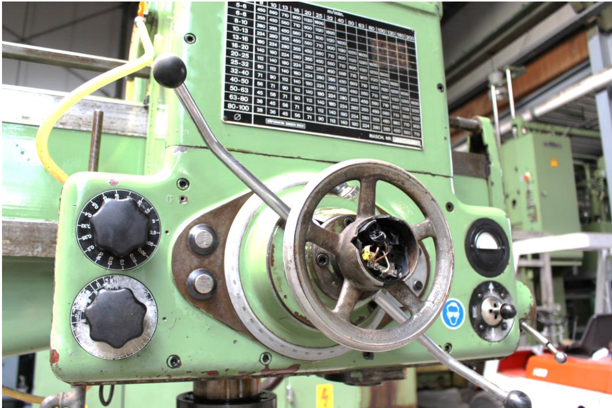
Die Schalteinheit zur Klemmung des Auslegers und des Bohrschlitten ist defekt
