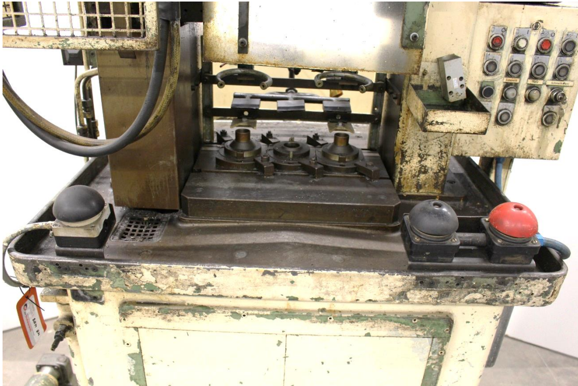
Maschinentisch mit 2 Hand Bedienung und Kühlschmiermitteleinrichtung
