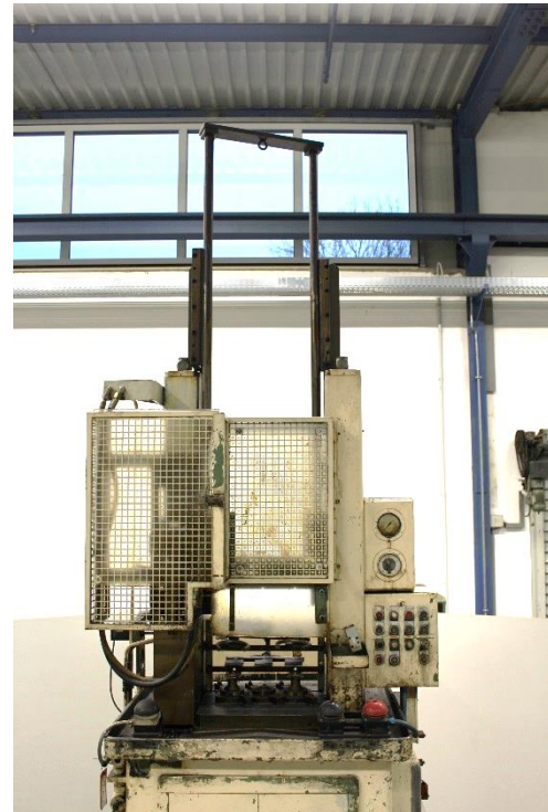
Bedienerumfeld mit Werkstücktisch und lang geführtem Werkzeug-Zubringerschlitten
