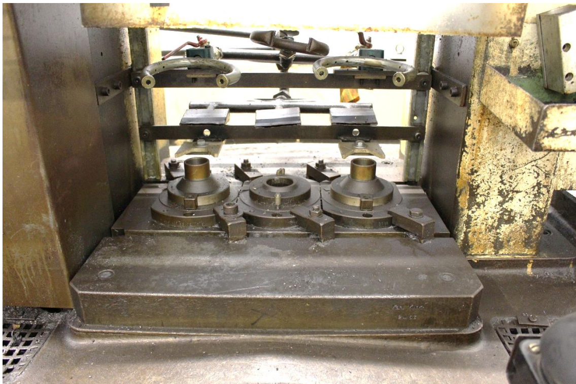
Maschinentisch für 3 Werkstücke
